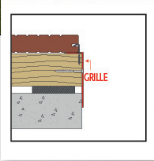
Exemple de grille de ventilation positionnée sous la lame
