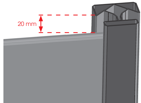
Schéma 4 : découpe du poteau
