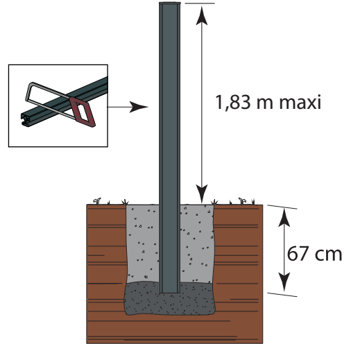
Schéma 3 : poteau à sceller
