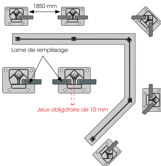
Schéma 1 : pose des poteaux
